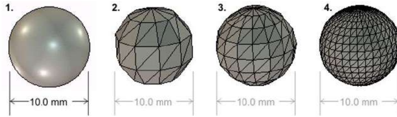
Şekil 4. STL formatındaki bir modelin üçgen yüzey geometrisi.
